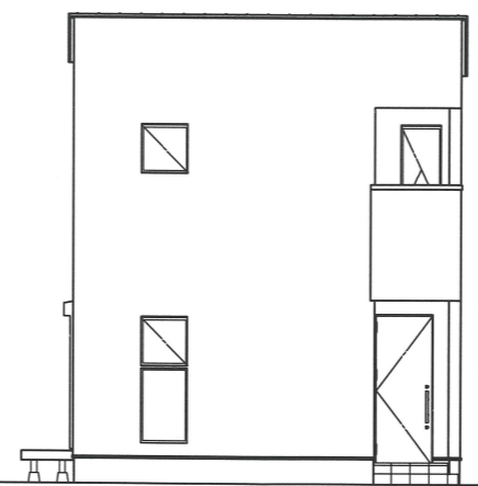
南側 立面図 S:1/130
